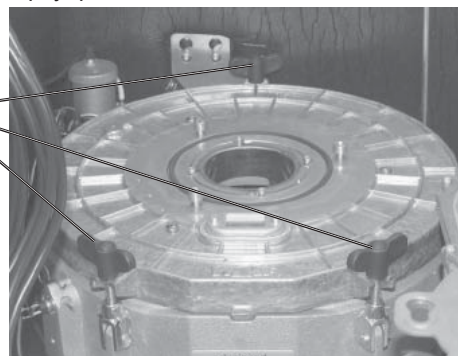
Барашковые винты
