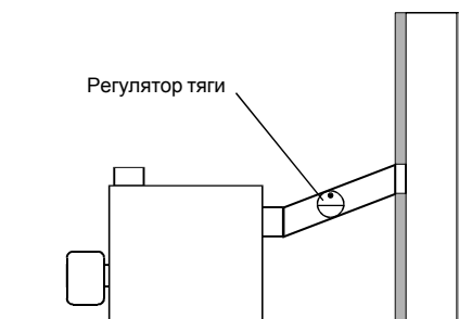
Рис. 4: Монтаж регулятора тяги в трубе для отвода отходящих газов
